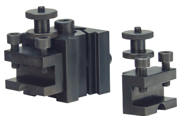
In dotazione una torretta portautensili multipla con 2 inserti.
